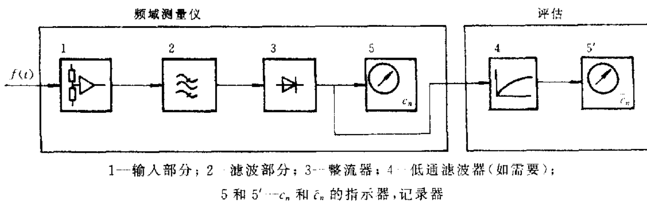
图 3 测量与评估测量仪器框图
