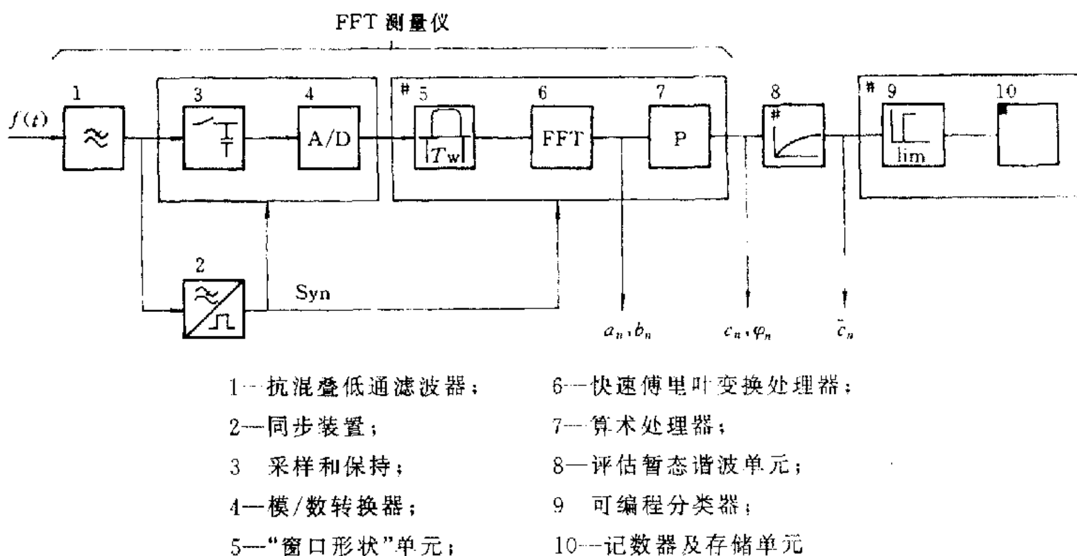
图 4 快速傅里叶变换测量仪框图(用于评估和分类)
